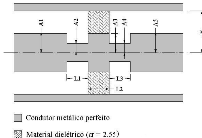
Figura 3.9 – Estrutura de acoplamento entre dois guias de onda coaxiais de dimensões iguais, utilizando carregamento dielétrico.
