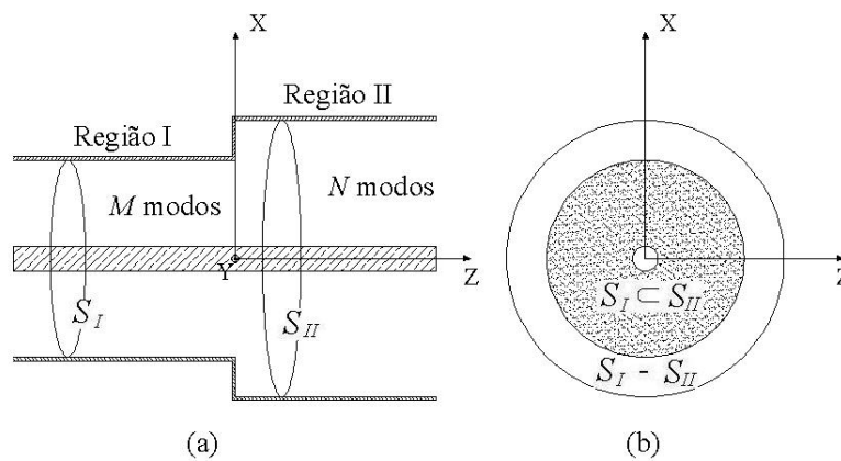
Figura 3.3 – Descontinuidade em guia de onda coaxial: (a) seção longitudinal e (b) seção transversal.
