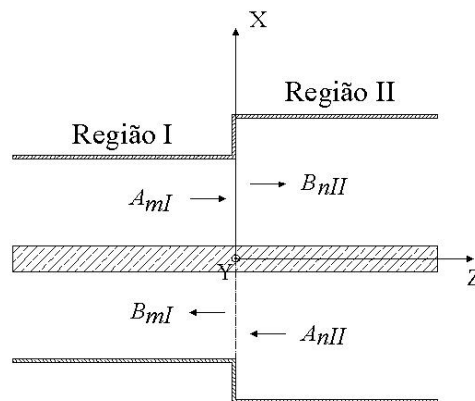
Figura 3.4 – Ilustração das amplitudes dos campos incidentes e espalhados na descontinuidades ( z = 0 ).
