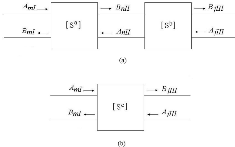
Figura 3.6 – (a) representação das duas matrizes de espalhamento conectadas, (b) representação da matriz de espalhamento geral obtida pelo cascadeamento.
