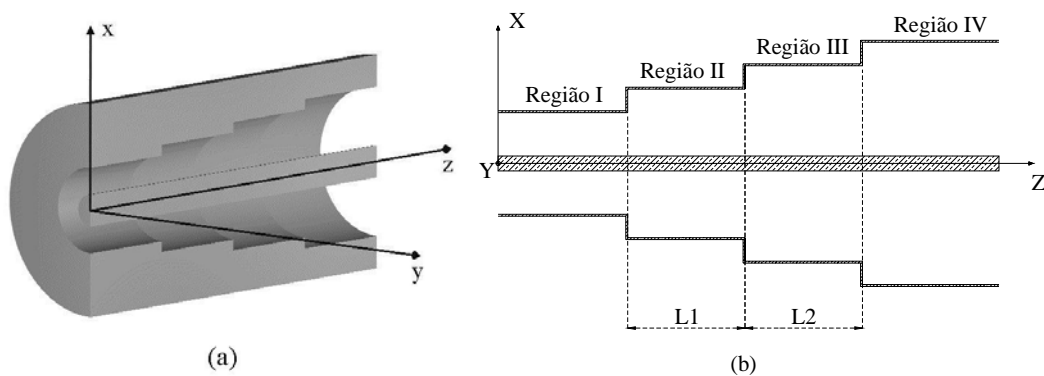
Figura 3.1 – Estrutura de acoplamento entre dois guias de onda coaxiais infinitos de dimensões arbitrárias. (a) Visão espacial e (b) seção longitudinal da estrutura de acoplamento.
