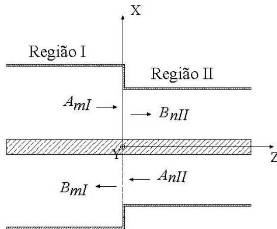
Figura 3.5 – Descontinuidade decrescente em guia de onda coaxial.
