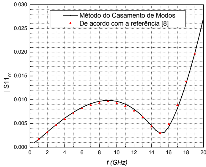
Figura 3.8 – |S11_{00}| (dB) para a estrutura de acoplamento da Figura 3.7.
