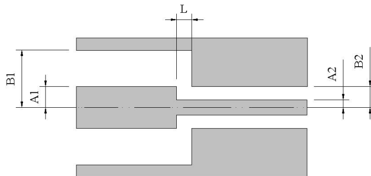
Figura 3.7 – Estrutura de acoplamento entre dois guias de onda coaxiais de dimensões distintas.
