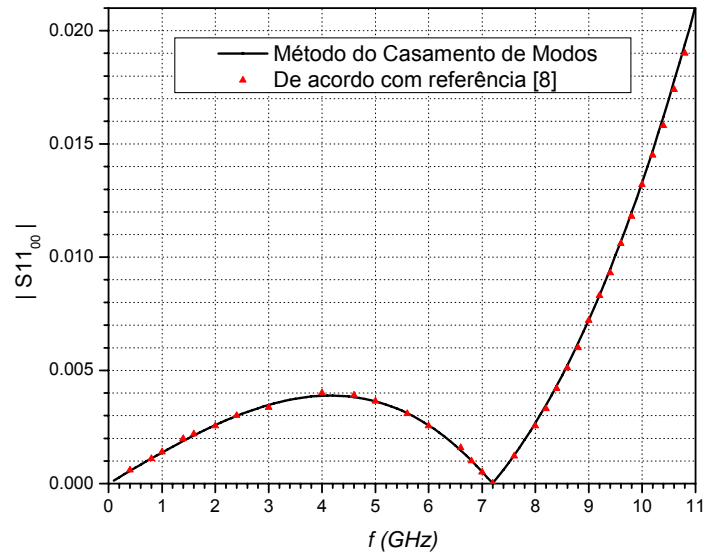
Figura 3.10 – |S_{11_{00}}| (dB) para a estrutura de acoplamento da Figura 3.9.
