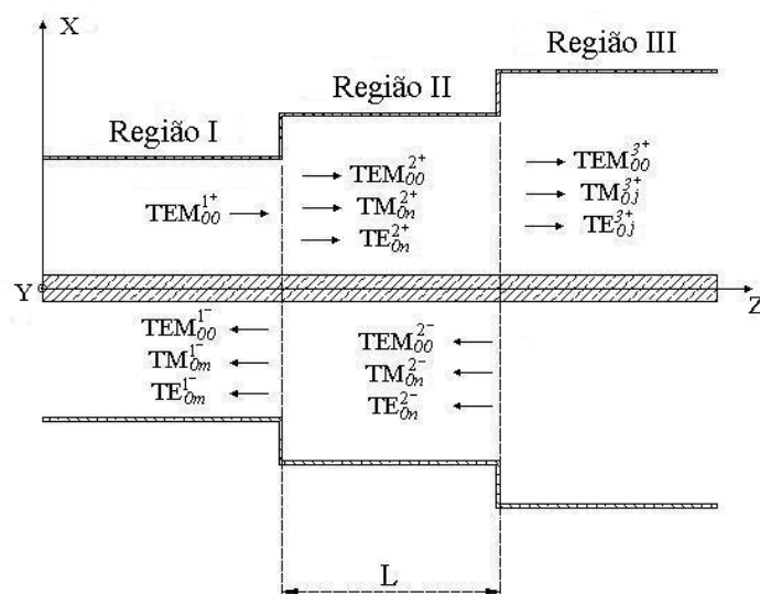
Figura 3.2 – Ilustração dos modos refletidos e transmitidos em cada descontinuidade de guia de onda coaxial.
