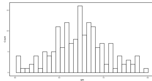
(b) SPI
