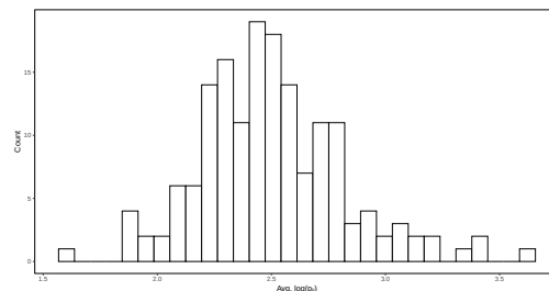
(d) \log(\bar{p}_i^{\text{geom}})
