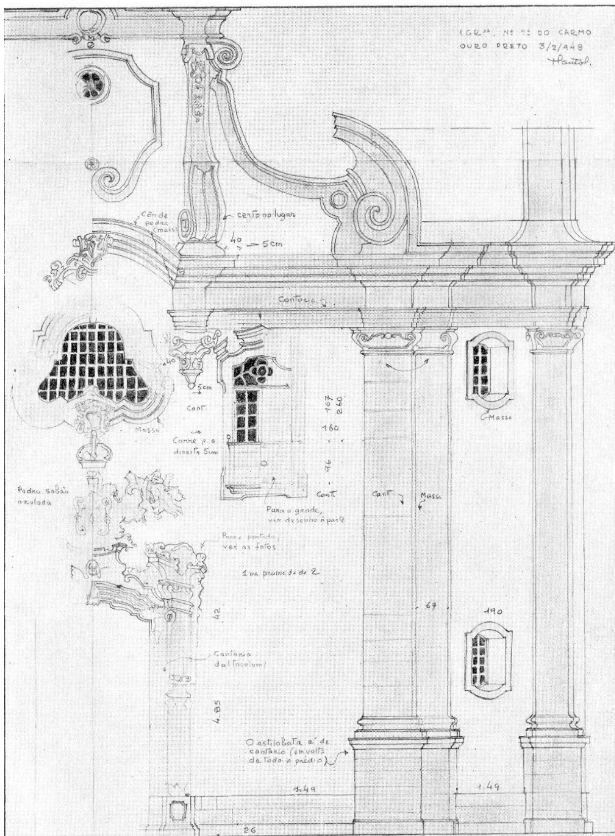
Croqui 7 Frontispício da Igreja de N. S.ª do Monte Carmo - Ouro Preto Levantamento e desenho: Paulo Ferreira Santos - 1949 Fonte: SANTOS, 1951a, fig. 150
