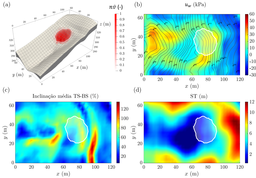
Figura 4.12: Resultados da simulação ( n_s=75 , \delta = 50 \text{ m} , 13 dias de chuva intensa): Escala de flutuação maior. (a) A visualização 3D mostra a zona de falha identificada (delimitada por uma linha branca contínua) com base no campo de velocidades normalizadas. (b) O gráfico 2D exhibe a distribuição da poro pressão na interface solo-rocha. Uma convenção de sinais negativos indica pressões de sucção. As linhas de contorno pretas contínuas representam a elevação ou depressão da rocha. (c) A vista superior 2D mostra a distribuição da inclinação média topográfica da rocha. (d) A vista superior 2D ilustra a distribuição da espessura da camada de solo.
