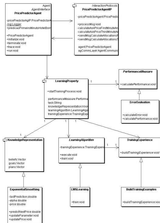
Figura 54: O diagrama de Classes (UML) do Preditor de Preços.
