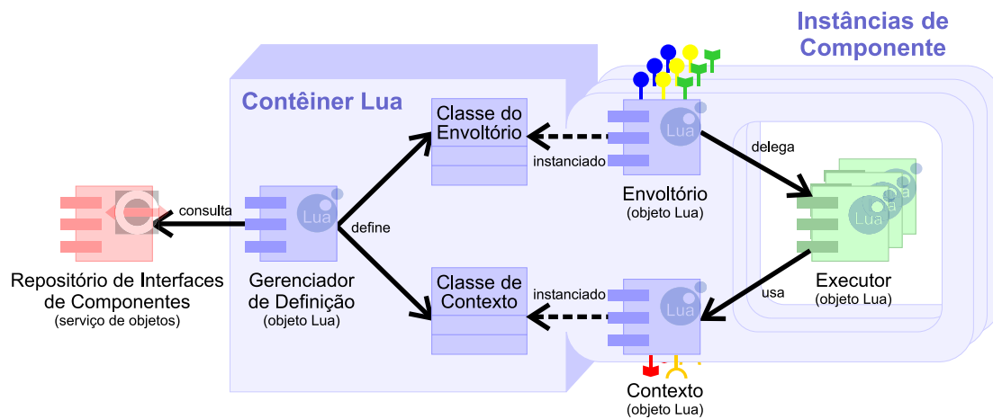
Figura 4.3: Arquitetura de gerência de definições de componentes do LuaCCM.
