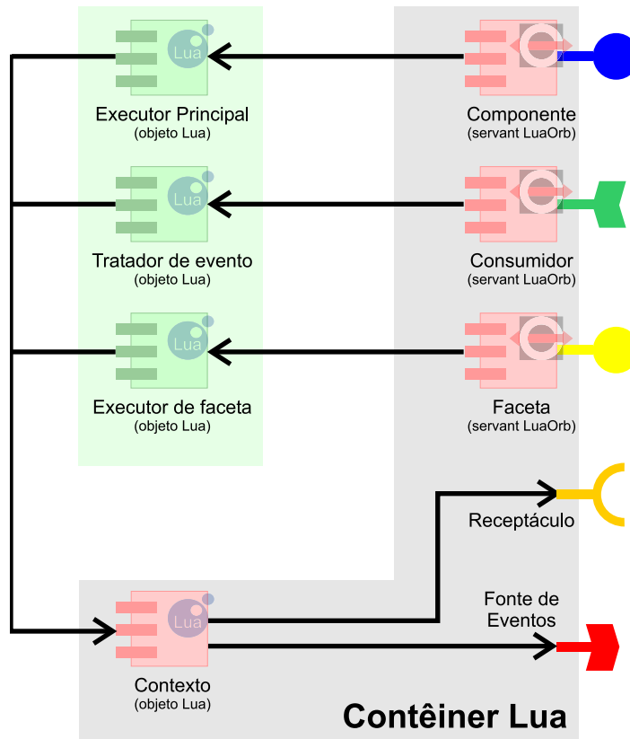
Figura 4.2: Estrutura do contêiner Lua.
