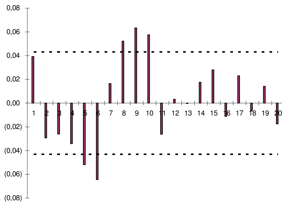
FIGURA 4.7 - PACF - IBV
