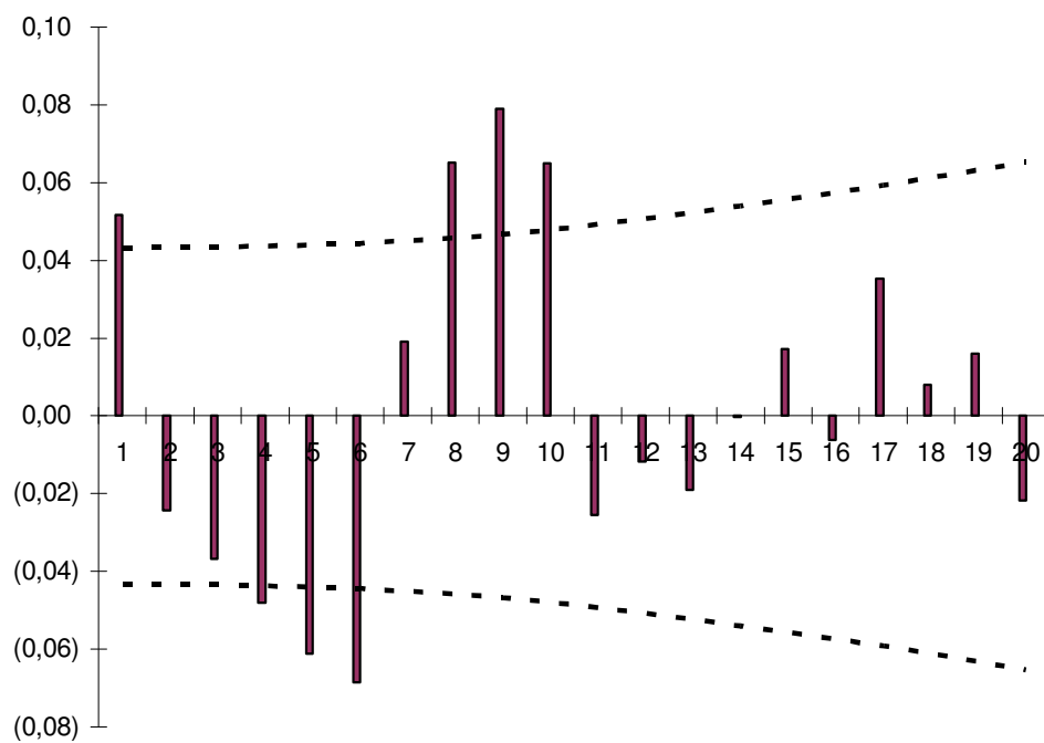
FIGURA 4.6 - ACF - IBV
