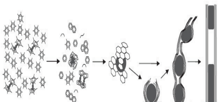
Figura 3.2: [Ref.[27]] Representação esquemática do mecanismo de crescimento para nanotubos de carbono produzidos por pirólise de hidrocarbonetos. Nela o material é craqueado na superfície da partícula metálica, podendo juntar-se à terminação de um tubo em formação dando continuidade ao crescimento.
