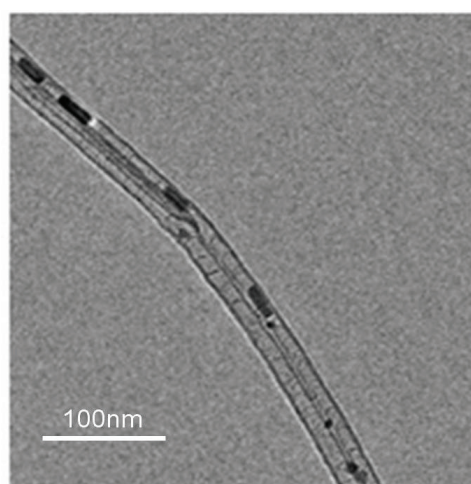
Figura 3.3: Imagem de microscopia de transmissão apresentando partículas metálicas no interior de nanotubos de carbono, indicando ser possível o processo de crescimento sugerido na ref.[27]. Essa é a amostra #06 setor C produzida com 100% de acetonitrila e temperatura 900°C.
