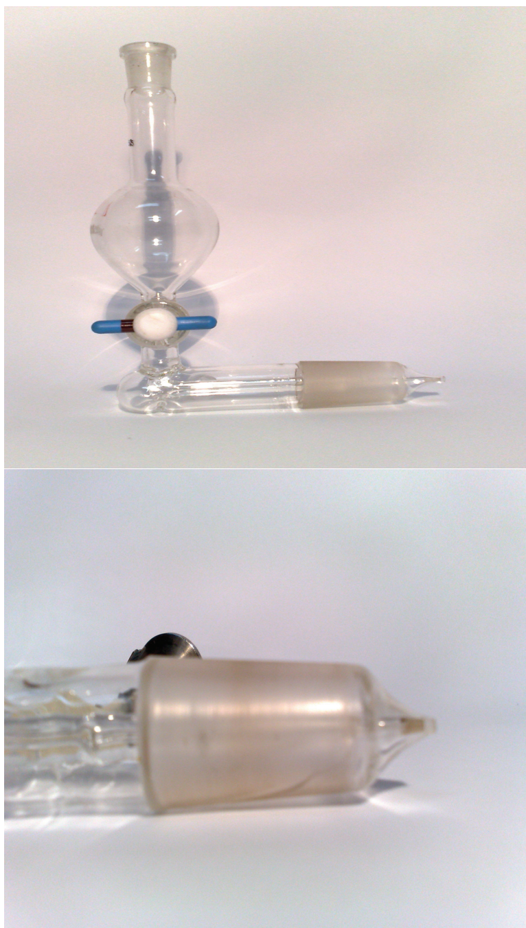
Figura 3.4: O Balão injetor. Essa é uma peça chave. Para uma deposição adequada o preciso ajuste dos diâmetros interno e externo do capilar interno e do bico de saída são responsáveis por permitir que a admissão do material se dê de forma adequada na região de deposição. Em baixo um detalhe do bico injetor.
