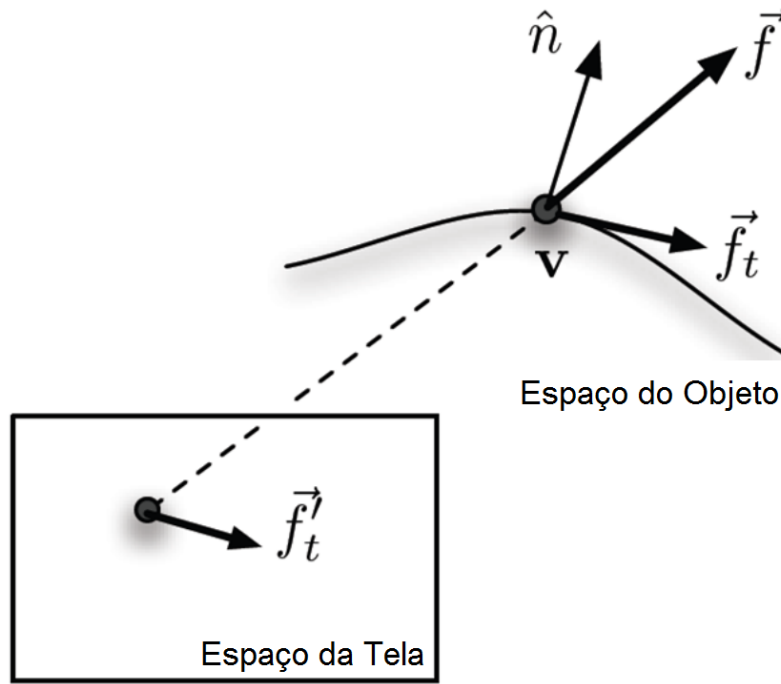
Figura 3.1: Projeção de um vetor do campo no espaço da tela.
