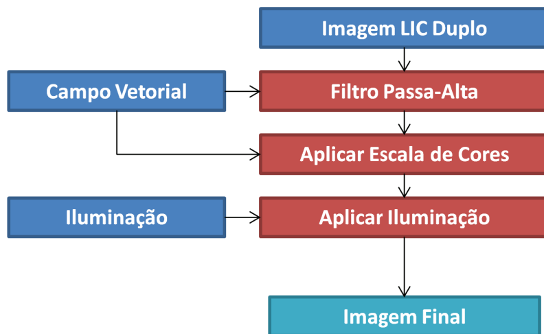
Figura 3.12: Etapa de Aplicação do Filtro Passa-Alta.
