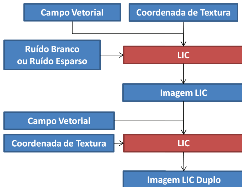
Figura 3.11: Etapa de Convolução por Integral de Linha.
