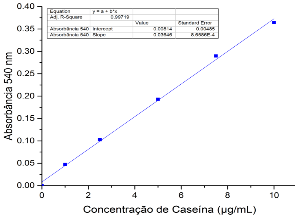
Figura 57. Curva padrão para proteínas.
