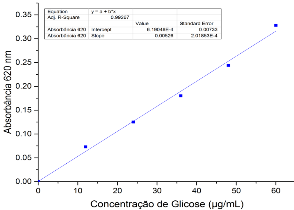
Figura 56. Curva padrão para carboidratos.
