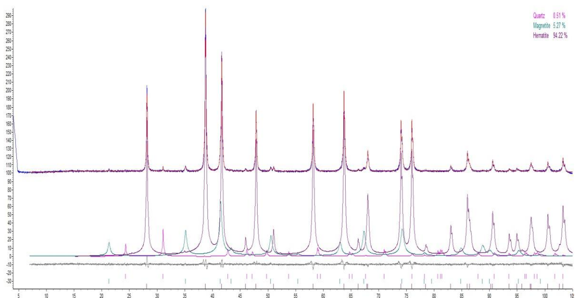
Figura 55. Difratoograma da amostra de hematita, tamanho (<math><20 \mu\text{m}</math>).
