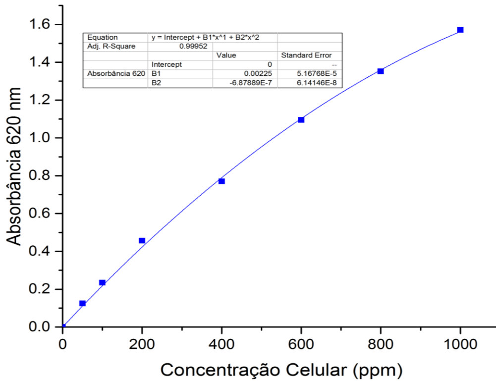
Figura 58. Curva de calibração da bactéria Rhodococcus erythropolis , relação entre concentração celular e absorvâncias.
