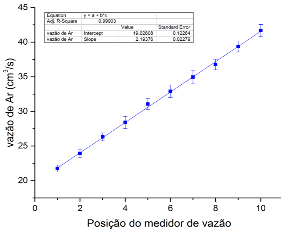
Figura 59. Curva de calibração do rotâmetro.
