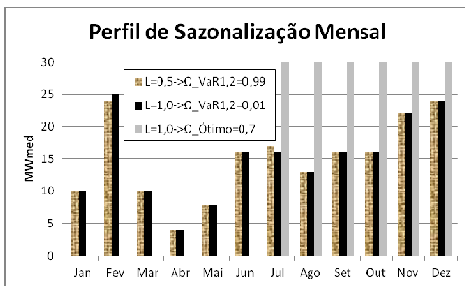
Figura 14 – Perfis de Sazonalização com \text{VaR}_{95\%} de R$1,2 milhão.
