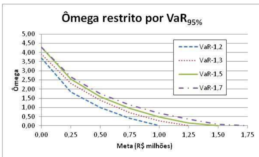
Figura 10 – Ômega restrito por VaR_{95\%} .
