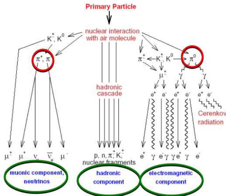
Figura 2.9: Componentes de um chuvaire atmosférico extenso (EAS).
