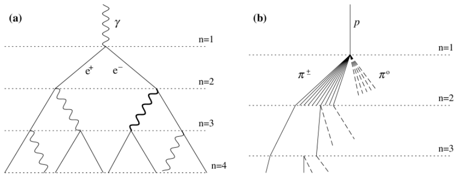
Figura 2.10: Chuvaire atmosféricos extensos segundo o Modelo de Heitler. a) chuvaire EM, b) chuvaire hadrônico. Extraída da referência [38].
