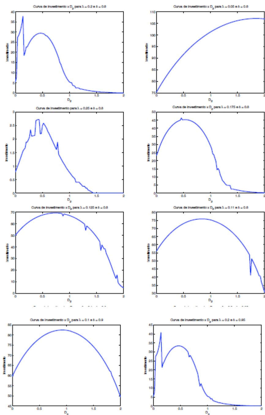
Figura 2.1: Curvas de investimento para diferentes combinações de \lambda e \delta
