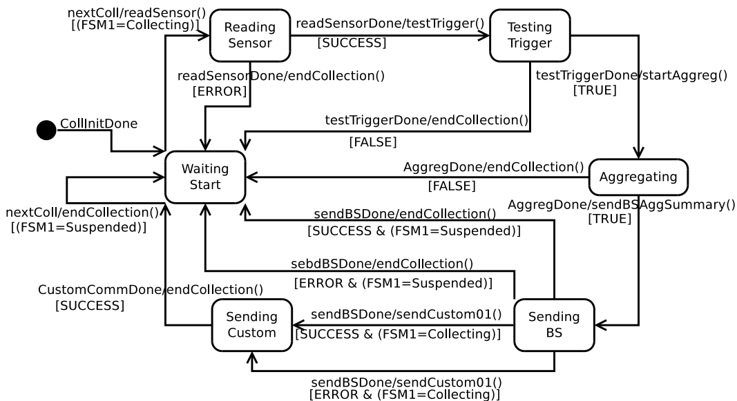
Figura 5.2: Aplicação 1 - FSM para geração do alarme
