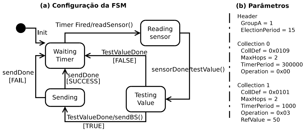
Figura 5.6: (a) FSM para controle de uma aplicação de alarme e (b) Definição dos respectivos parâmetros
