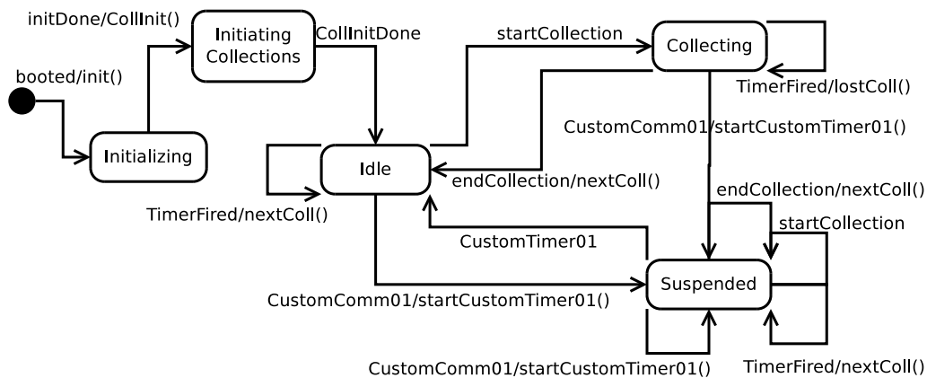
Figura 5.1: Aplicação 1 - FSM para inicialização do mote e controle geral da aplicação
