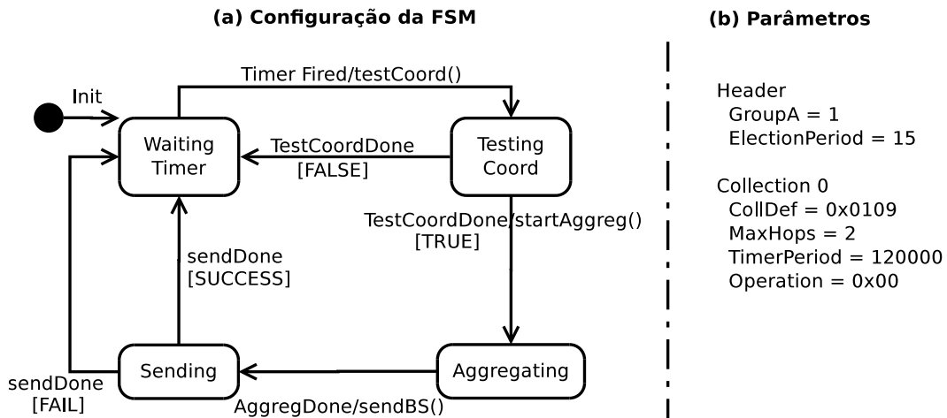
Figura 5.4: (a) FSM para controle de uma aplicação de coleta e (b) Definição dos respectivos parâmetros.
