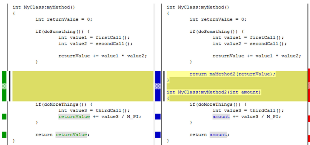
Figura 4 – Exemplo de comparação textual sobre duas versões de um documento onde um trecho de código é extraído para um novo método.
