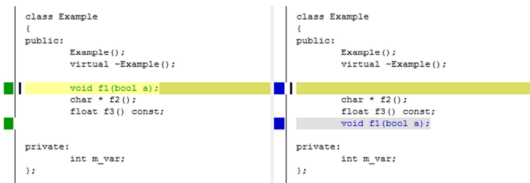
Figura 2 – Exemplo de comparação textual sobre duas versões de um documento onde a ordem das declarações é modificada.
