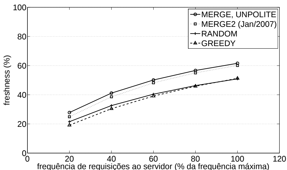
Figura 6.3: Freshness do repositório WIKIPEDIA após a execução das políticas MERGE, MERGE2, RANDOM e GREEDY, variando a frequência de requisições ao servidor.
